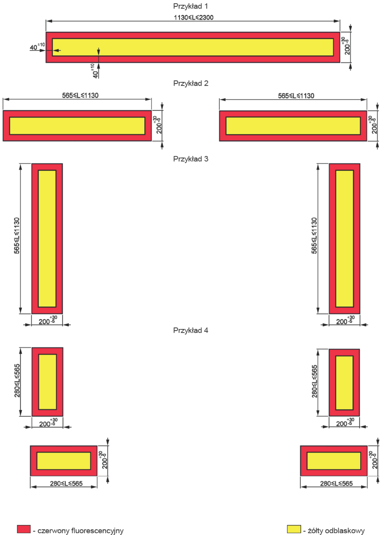
Rys. 2. Tablice wyróżniające przyczepę (naczepe) (mm)
